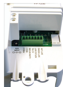
ONT Packet Cable Interface
